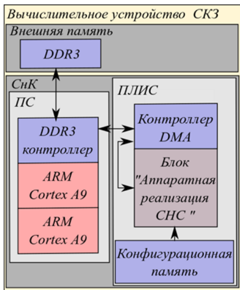
Рис. 2. Укрупненная функциональная схема ВУ Fig. 2. Enlarged functional diagram of the WU
