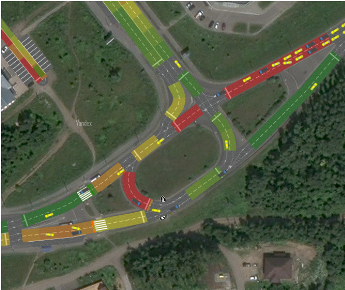
Рис. 4. Динамика дорожной ситуации после 120 минут моделирования. Цветовая схема на рисунке отражает среднюю скорость движения автомобилей на различных участках перекрёстка. Используются следующие обозначения: красный – до 10 км/ч; оранжевый – 10–20 км/ч; жёлтый – 20–30 км/ч; зелёный – более 40 км/ч
