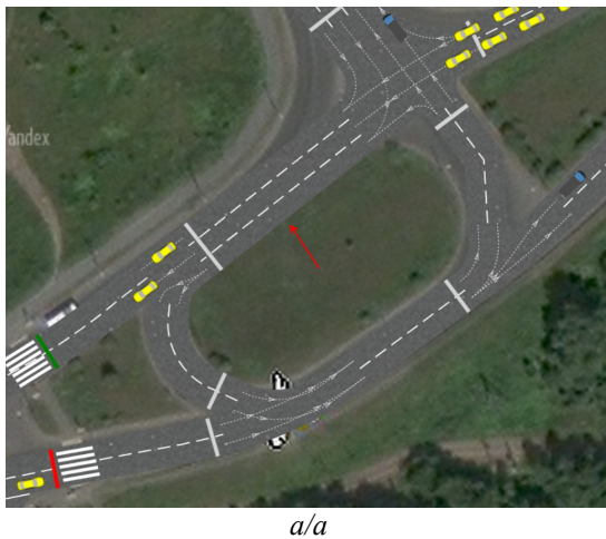
Рис. 6. Моделирование перекрёстка с увеличенной проезжей частью в одном из направлений: а) расположение дополнительной полосы; б) гистограмма времени пребывания агентов в пределах перекрёстка
