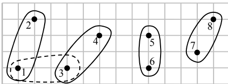
Рис. 1. Эффект обособления скоплений
