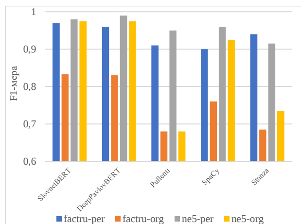
Рис. 2. Сравнение библиотек для извлечения именованных сущностей на наборах factru и ne5 для тегов личность (per) и организация (org)
