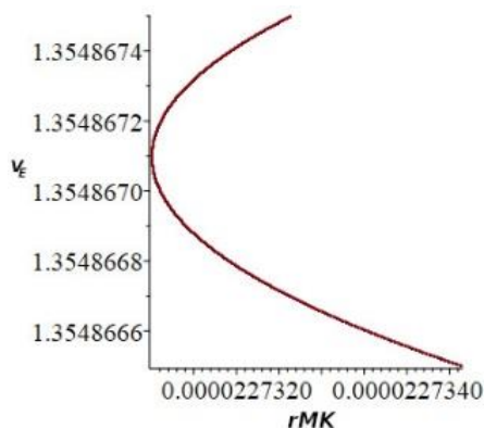
Рис. 8. Минимальное расстояние между космическим аппаратом и Марсом: r_{MK} \approx 0,000022731 а.е. – значение расстояния; v_E \approx 1,3548671 рад. – значение средней долготы Земли
