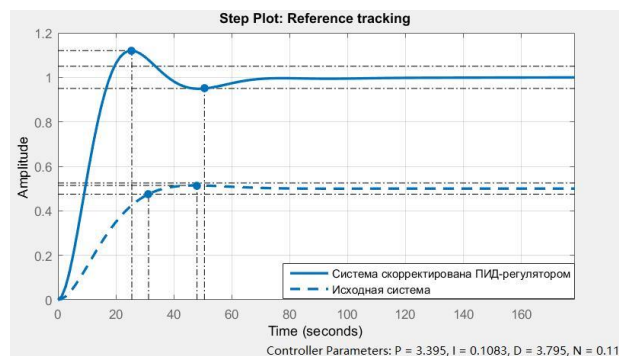
Рис. 4. Автоматическая настройка ПИД-регулятора в Simulink
