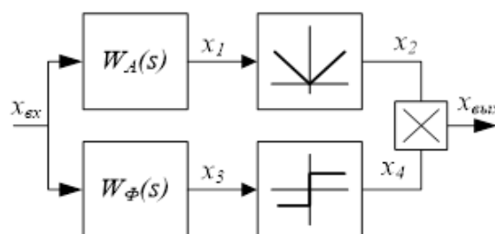
Рис. 1. Структурная схема корректирующего устройства с раздельными каналами для амплитуды и фазы
