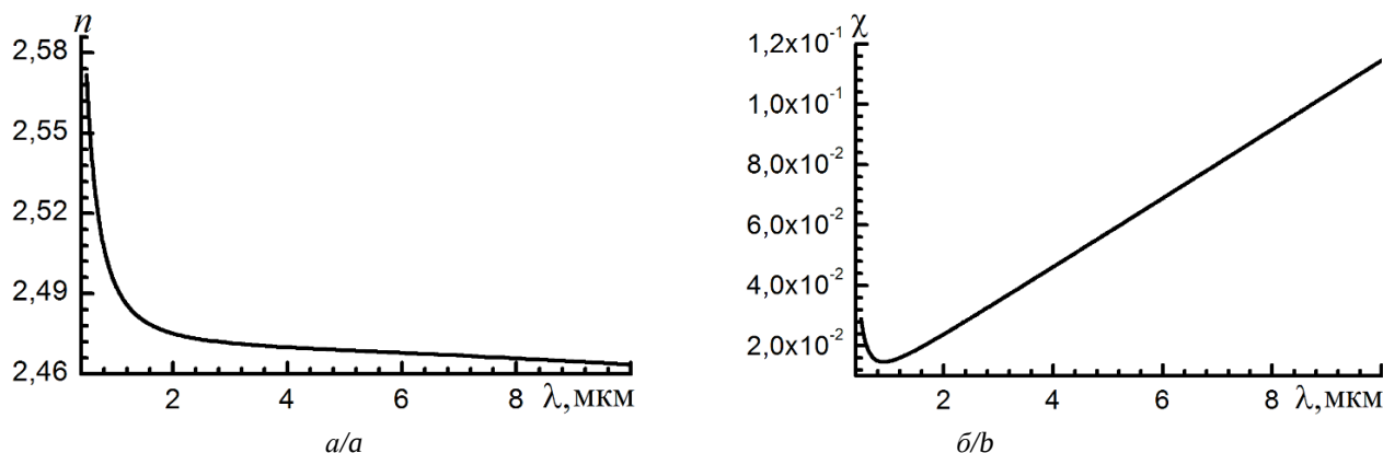
Рис. 2. Зависимости реальной n=n(\lambda) (а) и мнимой \chi=\chi(\lambda) (б) частей комплексного показателя преломления от длины волны для аморфного углерода [15]
