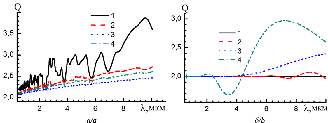
Рис. 6. Фактор ослабления Q(\lambda) для совокупности частиц аморфного углерода: а) для сфер при \mu=5 , \bar{a}=2 мкм (кривая 1), \mu=5 , \bar{a}=5 мкм (кривая 2), \mu=5 , \bar{a}=10 мкм (кривая 3), \mu=1 , \bar{a}=5 мкм (кривая 4); б) для пластинок при \mu=1 , \bar{a}=40 мкм, d=2,020 \cdot (2 \cdot a)^{0.449} (кривая 1), \mu=10 , \bar{a}=40 мкм, d=2,020 \cdot (2 \cdot a)^{0.449} (кривая 2), \mu=1 , \bar{a}=40 мкм, d=a/20 (кривая 3), \mu=10 , \bar{a}=40 мкм, d=a/20 (кривая 4)
