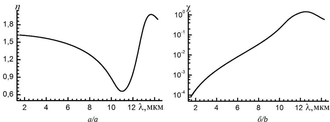
Рис. 3. Зависимости реальной n=n(\lambda) (а) и мнимой \chi=\chi(\lambda) (б) частей комплексного показателя преломления от длины волны для триоксида диалюминия [16, 17]
