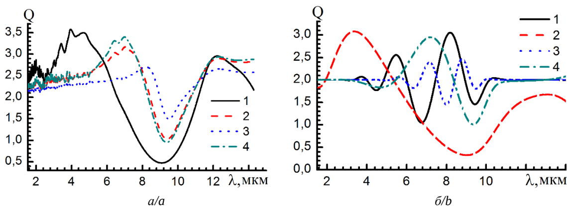
Рис. 7. Фактор ослабления Q(\lambda) для совокупности частиц триоксида диалюминия: а) для сфер при \mu=5 , \bar{a}=2 мкм (кривая 1), \mu=5 , \bar{a}=5 мкм (кривая 2), \mu=5 , \bar{a}=10 мкм (кривая 3), \mu=10 , \bar{a}=5 мкм (кривая 4); б) для пластинок при \mu=5 , \bar{a}=40 мкм, d=2,020 \cdot (2 \cdot a)^{0.449} (кривая 1), \mu=5 , \bar{a}=40 мкм, d=a/20 (кривая 2), \mu=5 , \bar{a}=140 мкм, d=2,020 \cdot (2 \cdot a)^{0.449} (кривая 3), \mu=5 , \bar{a}=140 мкм, d=a/20 (кривая 4)
