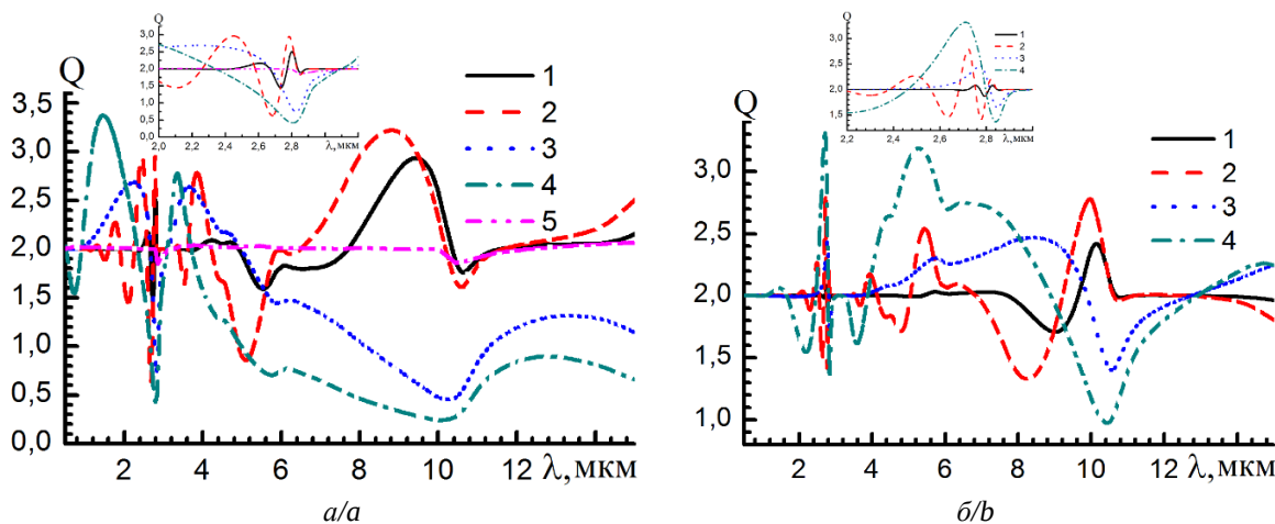
Рис. 5. Фактор ослабления Q(\lambda) для совокупности ледяных частиц: а) для пластинок \mu=1 , \bar{a}=40 мкм, d=2,020 \cdot (2 \cdot a)^{0,449} (кривая 1), \mu=10 , \bar{a}=40 мкм, d=2,020 \cdot (2 \cdot a)^{0,449} (кривая 2), \mu=1 , \bar{a}=40 мкм, d=a/20 (кривая 3), \mu=10 , \bar{a}=40 мкм, d=a/20 (кривая 4), для смеси 8 типов кристаллов при a_{\text{eff}}=40 мкм (кривая 5); б) для пластинок \mu=1 , \bar{a}=140 мкм, d=2,020 \cdot (2 \cdot a)^{0,449} (кривая 1), \mu=10 , \bar{a}=140 мкм, d=2,020 \cdot (2 \cdot a)^{0,449} (кривая 2), \mu=1 , \bar{a}=140 мкм, d=a/20 (кривая 3), \mu=10 , \bar{a}=140 мкм, d=a/20 (кривая 4)
