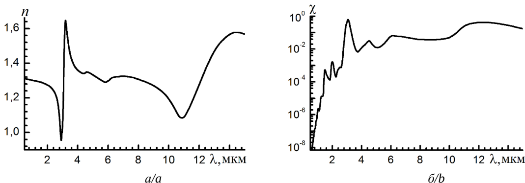
Рис. 1. Зависимости реальной n=n(\lambda) (а) и мнимой \chi=\chi(\lambda) (б) частей комплексного показателя преломления от длины волны для чистого льда [14]
