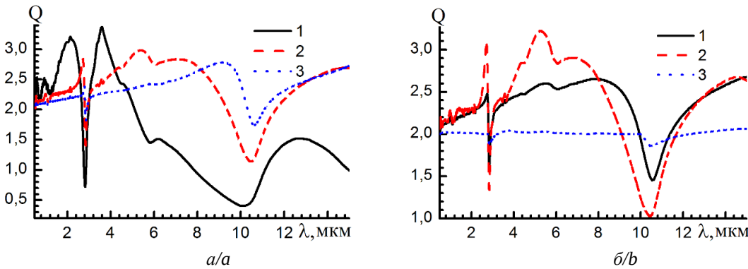
Рис. 4. Фактор ослабления Q(\lambda) для совокупности ледяных частиц: а) для сфер при \mu=5 : \bar{a}=2 мкм (кривая 1), \bar{a}=5 мкм (кривая 2), \bar{a}=10 мкм (кривая 3); б) для сфер при \bar{a}=5 мкм, \mu=1 (кривая 1), для сфер при \bar{a}=5 мкм, \mu=10 (кривая 2), для смеси 8 типов кристаллов при a_{\text{iff}}=5 мкм (кривая 3)
