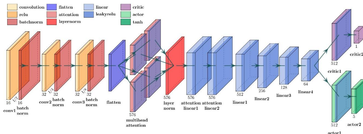
Рис. 6. Топология нейронной сети агента PPOv4
