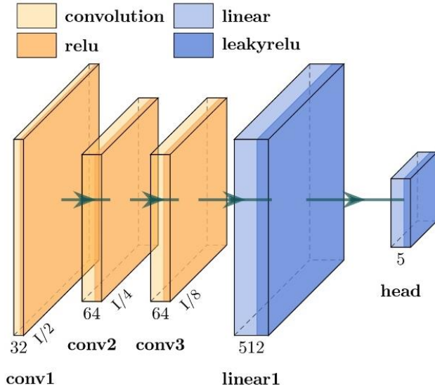
Рис. 2. Топология нейронной сети агента DQN Fig. 2. Topology of the neural network of the DQN agent
