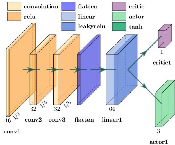
Рис. 3. Топология нейронной сети агента PPO Fig. 3. Topology of the neural network of the PPO agent
