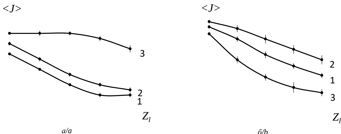
Рис. 6. Зависимость критерия фокусировки от длины трассы при задании искажений рядом полиномов Цернике (а) и фазовым экраном, моделирующим атмосферную турбулентность (б). Номера кривых соответствуют параметрам задачи, указанным в подписи к рис. 5
