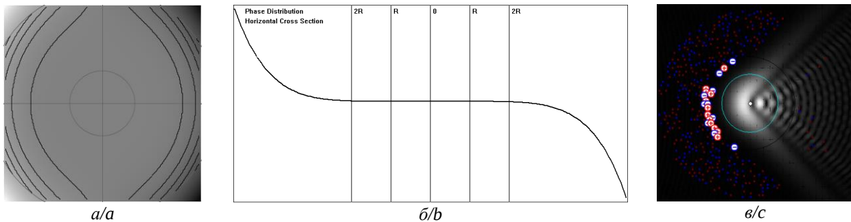
Рис. 1. Начальный фазовый профиль пучка (а), заданный полиномом № 7 (кома), изгиб поверхности показан полутоннами и линиями равного уровня; б) поперечное сечение фазового профиля; в) распределение амплитуды излучения (с указанными на нем вихрями), зарегистрированное на расстоянии Z=0,1 Fig. 1. Initial phase profile of the beam (a), given by polynomial No. 7 (coma), the surface bending is shown by halftones and equal-level lines; (b) cross-section of the phase; (c) distribution of radiation amplitude with the vortices indicated on it, recorded at a distance of Z=0.1
