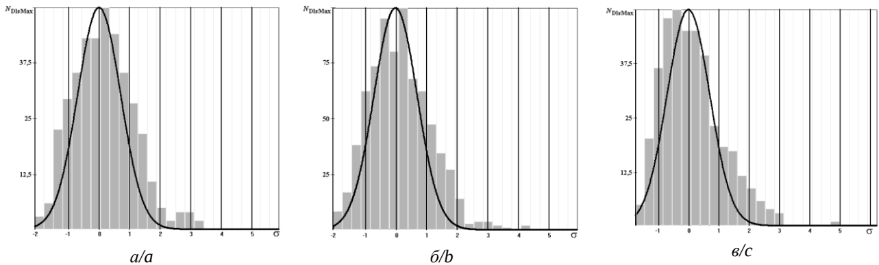
Рис. 4. Гистограммы случайного распределения оптических вихрей, иллюстрирующие выполнение центральной предельной теоремы. Сплошная линия – гауссова функция, соответствующая распределению. Число реализаций случайного процесса: а) 400; б) 800; в) 400. Фазовые искажения задаются экраном, моделирующим турбулентность (а, б) и рядом полиномов Цернике (в). N_{DiskMax} – число вихрей в одном интервале гистограммы
