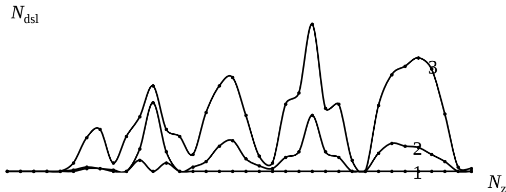
Рис. 2. Количество особых точек N_{dsl} в пучке при задании начальной фазы различными полиномами. N_z – номер полинома, a_i=1 , Z=0,1 . Кривая 1 получена при регистрации вихрей в области с диаметром равным начальному диаметру пучка; 2 – диаметр был увеличен до 1,2; 3 – до 1,4 начального диаметра Fig. 2. Number of special points N_{dsl} in the beam, when the initial phase is specified by different polynomials. N_z is the polynomial number, a_i=1 , Z=0.1 . Curve 1 was obtained when registering vortices in a region with a diameter equal to the initial diameter of the beam; 2 – the diameter was increased to 1.2; 3 – to 1.4 of the initial diameter
