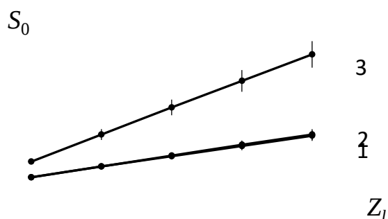
Рис. 8. Смещение энергетического центра пучка. Номера кривых соответствуют параметрам задачи, указанным в подписи рис. 5
