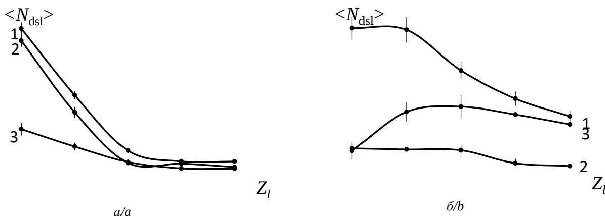
Рис. 5. Зависимость среднего числа \langle N_{dsl} \rangle зарегистрированных особых точек от длины трассы Z . Параметры задачи: а) ряд включает 30 (кривая 1), 20 (кривая 2) и 10 (кривая 3) полиномов. При задании фазы экраном, моделирующим атмосферную турбулентность, радиус Фрида и внутренний масштаб принимают следующие значения: б) r_0=0,6 , l_0=0,08 (кривая 1); r_0=0,6 , l_0=2 (кривая 2); r_0=0,2 , l_0=2 (кривая 3). Усреднение выполняется по 300 реализациям
