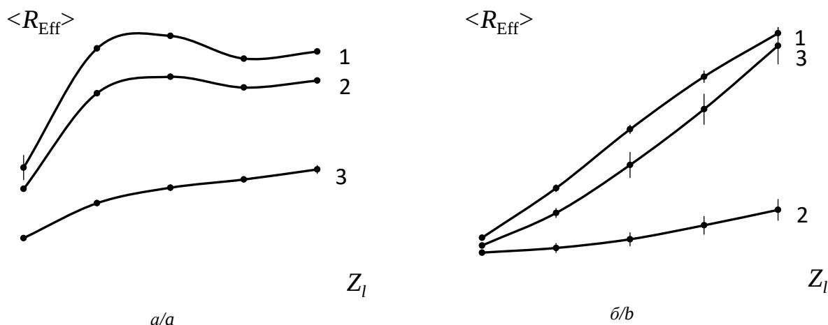
Рис. 7. Зависимость средних значений энергетического радиуса пучка от длины трассы. Номера кривых соответствуют параметрам задачи, указанным в подписи рис. 5
