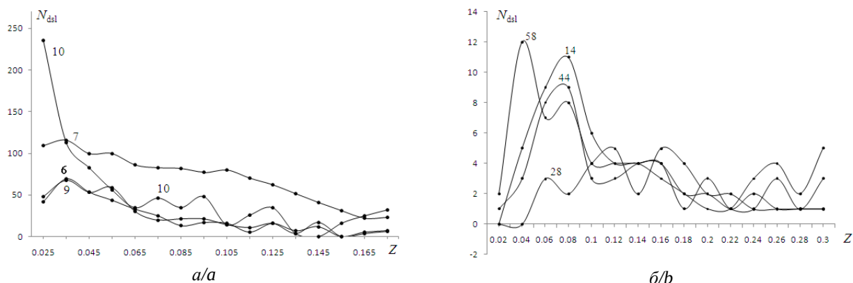
Рис. 3. Зависимость количества вихрей от длины трассы при задании фазы полиномами (а) и экраном, моделирующим турбулентность (б). а) указаны номера полиномов (кома, уравнение 3 и кома с поворотом на 90^\circ , трилистник, уравнение 4 и трилистник с поворотом на 90^\circ ), формирующих начальную фазу (нумерация OSA); б) номера случайных экранов (числа, являющиеся основанием при работе генератора случайных чисел), r_0=0,6
