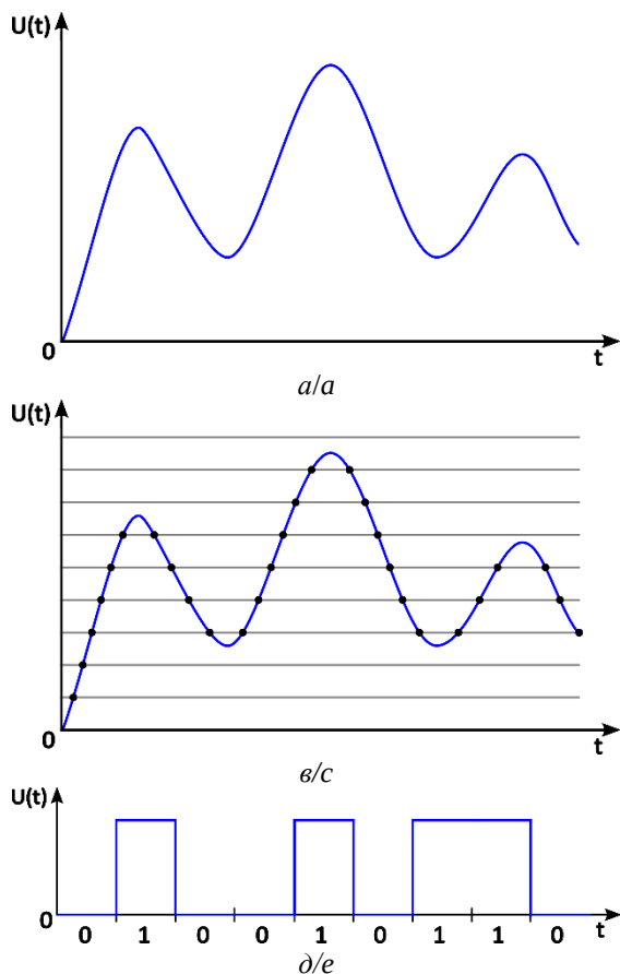
Рис. 1. Пример графика: а) аналогового сигнала; б) дискретного сигнала; в) квантованного сигнала; г) цифрового сигнала; д) двоичного цифрового сигнала
