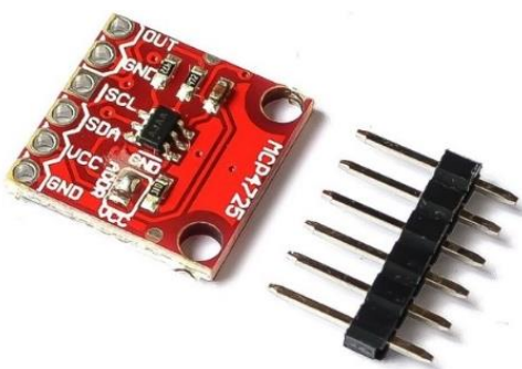
Рис. 2. Модуль ЦАП на микросхеме МСР4725 с интерфейсом I2C
