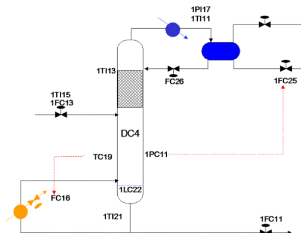
Рис. 1. Структурная схема колонны выделения бутана Fig. 1. Structural diagram of the butane extraction column
