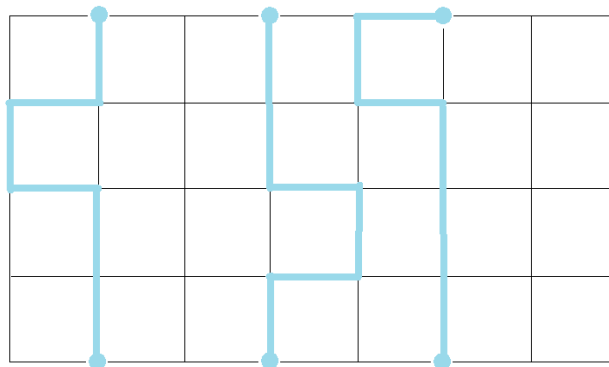
Рис. 8. Топология T2: вариант прокладки вторичной сети без совместного использования ветвей первичной
