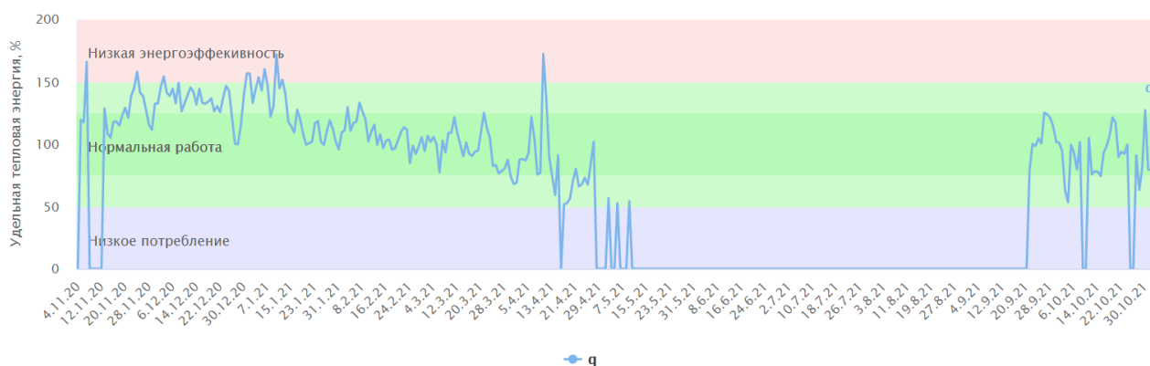
Рис. 6. График относительного удельного теплоснабжения рассматриваемой системы здания Fig. 6. Graph of the relative specific heat consumption of the building system under consideration
