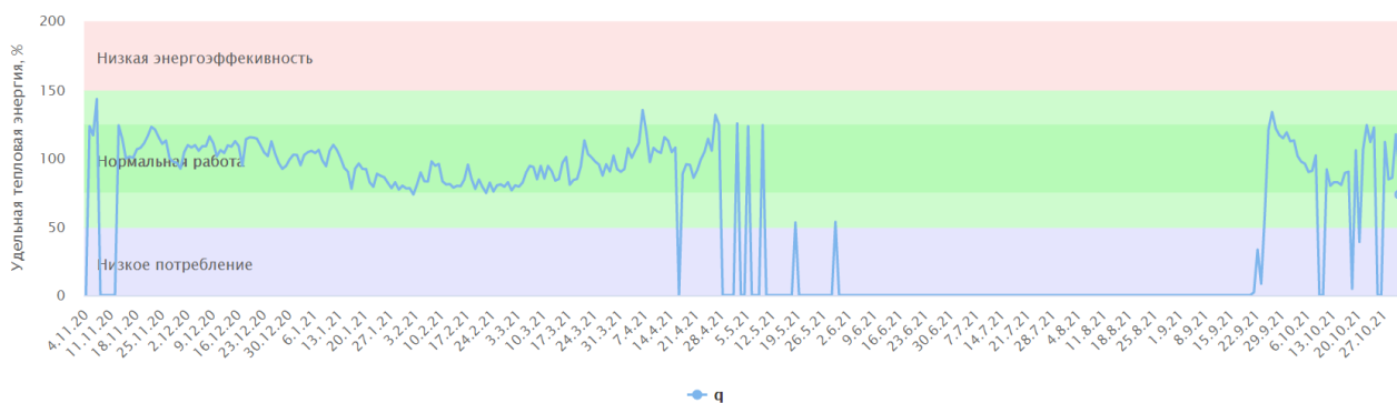
Рис. 7. График относительного удельного теплоснабжения системы альтернативного здания Fig. 7. Graph of relative specific heat consumption of an alternative building system
