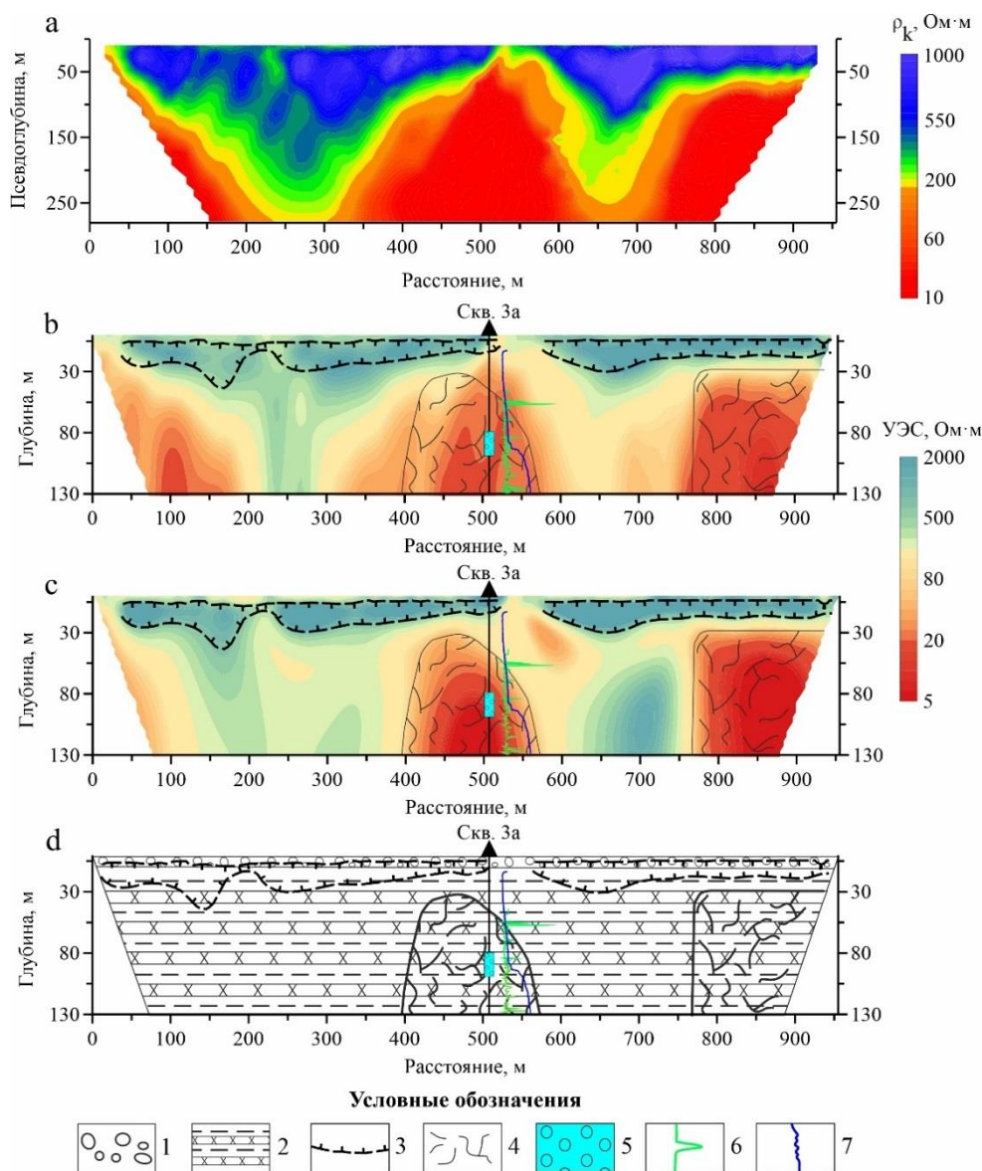
Рис. 6. Разрезы по профилю № 5: а) по параметру кажущегося сопротивления; б) по параметру УЭС на основе решения одномерной обратной задачи электроразведки; в) по параметру УЭС на основе решения двумерной обратной задачи электроразведки; д) схематический геологический разрез, составленный по данным бурения. 1 – валунно-галечные отложения; 2 – переслаивание аргиллитов и алевролитов; 3 – зона ММП; 4 – зона трещиноватости; 5 – обводненный интервал; 6 – кривая каротажа сопротивления; 7 – кривая термометрии
