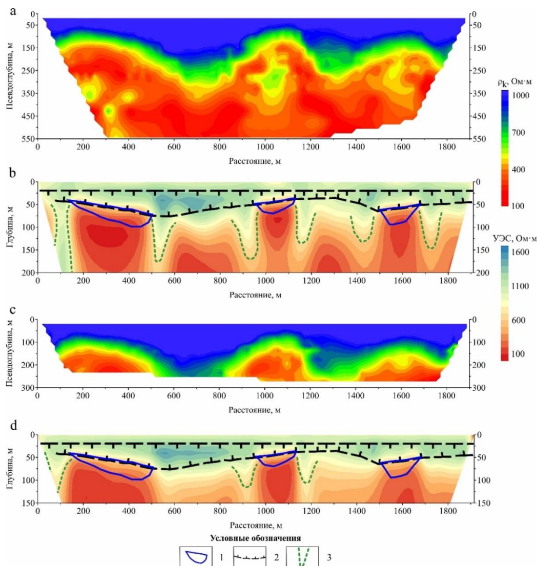
Рис. 5. Результаты решения прямой и обратной задачи электроразведки для трехэлектродной установки с шагом 5 м (а и б соответственно) и 10 м (с и д соответственно) для модели А: 1 – контур таликовых зон; 2 – зона ММП; 3 – высокоомные субвертикальные структуры, оконтуривающие таликовые зоны
