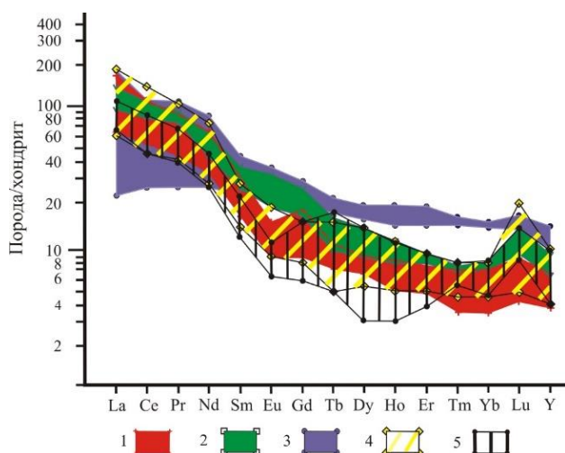
Рис. 4. Спайдер-диаграмма распределения редкоземельных элементов в породах и рудах Амзарканского месторождения. Поля на диаграмме: амуджиканский интрузивный комплекс (J2-3): 1 – гранодиориты, 2 – диориты; 3 – базальты нюкжинской серии (J3); рудоносные жилы: 4 – сульфидно-кварцевые, 5 – сульфидно-кварцевые с включениями графита
