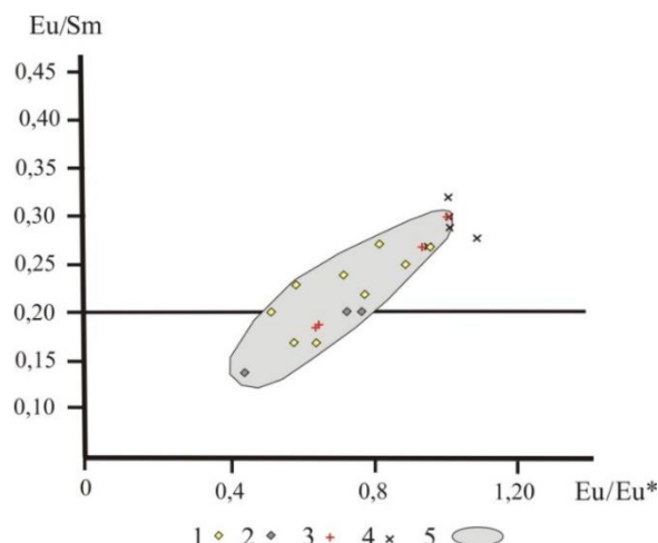
Рис. 5. Диаграмма Eu/Sm-Eu/Eu^* интрузивных и рудных образований Амзарканского месторождения. Значения: 1 – сульфидно-кварцевые руды, 2 – кварцево-графитовые жилы; амуджиканский комплекс: 3 – гранодиориты, 4 – диориты; 5 – область значений распределения рудных жил и гранодиоритов амуджиканского комплекса
