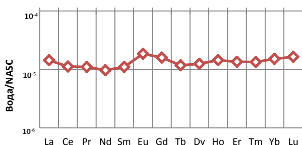
Рис. 11. Распределение содержания редкоземельных элементов в пробе конденсационной влаги, собранной на отвале № 2 Ермаковского месторождения, нормированных по отношению к содержанию в NASC
