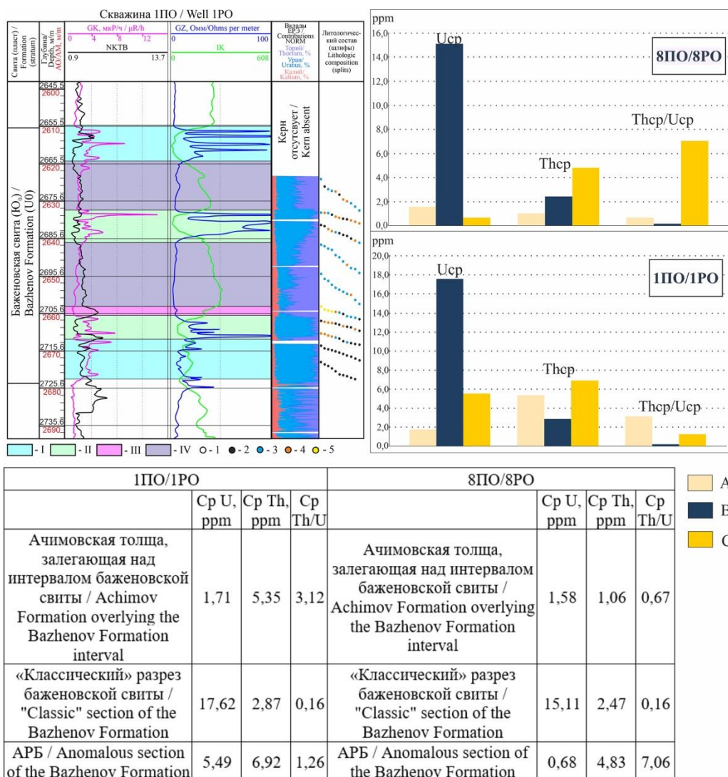
Рис. 2. Дифференциация баженовской свиты по данным исследования керна и распределение естественной радиоактивности (ЕРЭ) (Литогеохимические интервалы: I – преобладающе кремниевый состав, II – преобладающе кремниво-карбонатного состава, III – терригенного состава песчано-алевритовой размерности, IV – терригенного состава глинистой размерности. Литогеохимический состав в шлифах: 1 – место отбора шлифа, 2 – преимущественно кремниевый состав, 3 – преимущественно терригенный состав глинистой размерности, 4 – преимущественно карбонатный состав, 5 – преимущественно терригенный состав песчано-алевритовой размерности. Распределение ЕРЭ: А – ачимовская толща, В – карбонатно-кремневая часть баженовской свиты, С – терригенная часть баженовской свиты)
