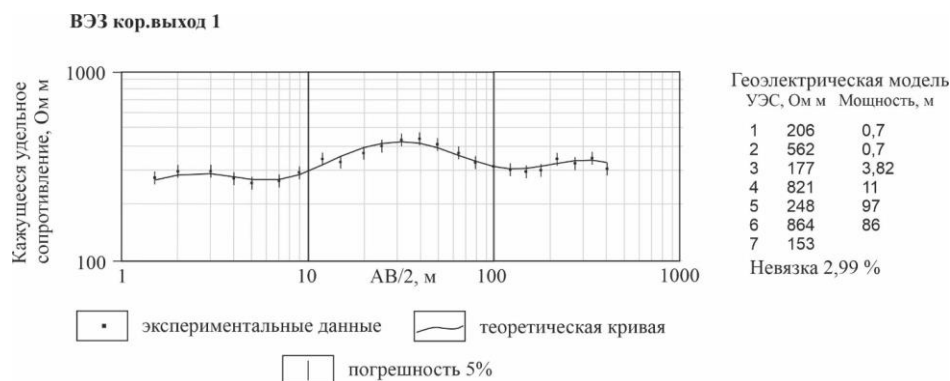
Рис. 6. Кривая ВЭЗ и геоэлектрическая модель
