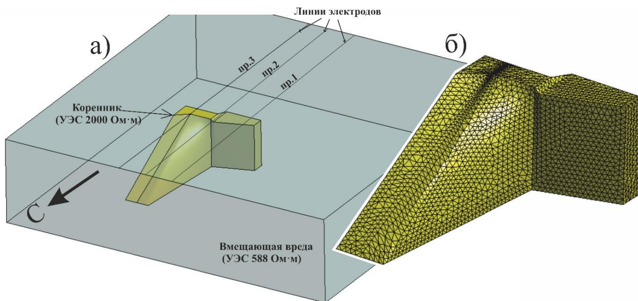
Рис. 3. а) модель № 1, построенная в программе GiD; б) фрагмент объекта-коренника с тетраэдральной сетью разбиения с мелкостью 5
