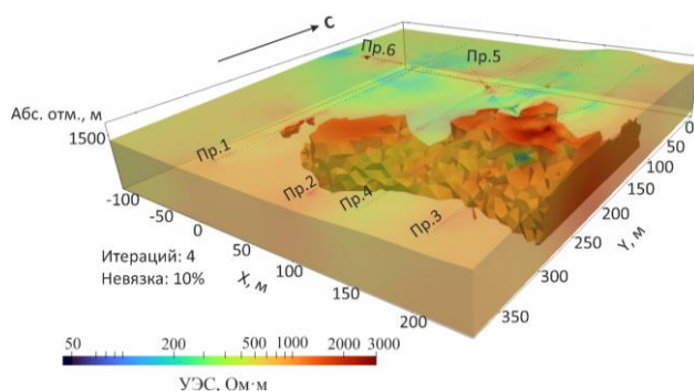
Рис. 2. 3D-инверсия полевых данных
