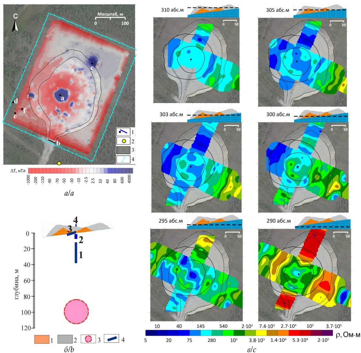
Рис. 11. Магнитные аномалии (нТл) (а), схема предположительного расположения фрагментов обсадной колонны боевой скважины (№ 1–3) и столба-репера (№ 4) (б) и распределение УЭС на разной глубине (Ом·м) (в) на эпицентре ПЯВ «Кристалл». Черным штрихом показаны подножье и верхняя кромка насыпи, черной жирной линией – подножье и гребень навала. Условные обозначения (а): 1 – железные объекты на поверхности: а) столб-репер; б) две трубы под насыпной дорогой; в) шина карьерного грузовика БЕЛАЗ; г) бочки; д) лист; е) проволока; 2 – магнитовариационная станция; 3 – центральная магнитная аномалия; 4 – забор; (б): 1 – навал; 2 – насыпь; 3 – центральная зона взрыва; 4 – железные объекты
