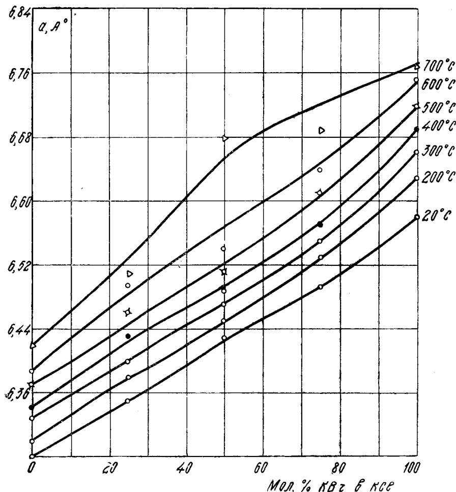
Рис. 1. Изменение периода решетки твердых растворов \text{KCl}-\text{KBr} в зависимости от состава при высоких температурах.
