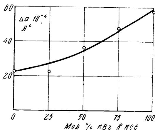
Рис. 4. Зависимость изменения периода решетки \Delta a от состава твердого раствора KCl—KBr.
