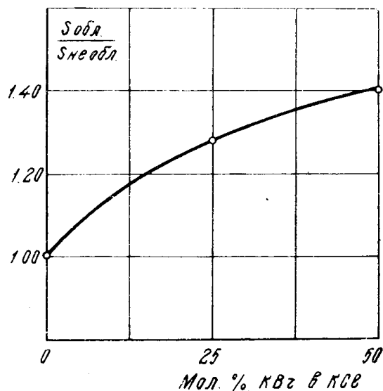
Рис. 3. Зависимость отношения \frac{S_{obl}}{S_{neobl}} от состава твердого раствора KCl—KBr.
