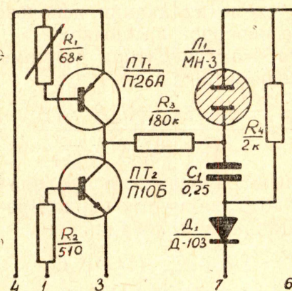
Рис. 10. Принципиальная схема модуля ЭР-2.
