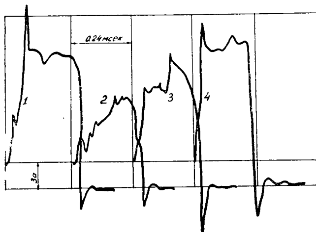
Рис. 2. Кривые тока коммутации в продольной цепи при токе нагрузки 5,3 \text{ а} и частоте 50 \text{ гц} .
