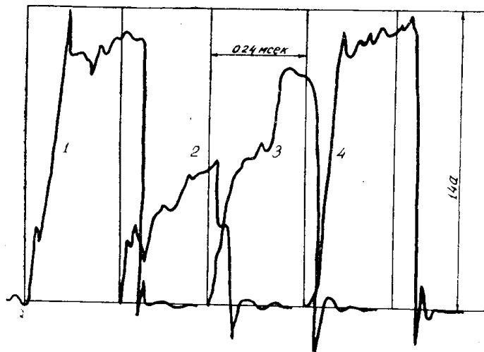
Рис. 1. Кривые тока коммутации в продольной цепи при холостом ходе усилителя и частоте 50 \text{ гц} .
