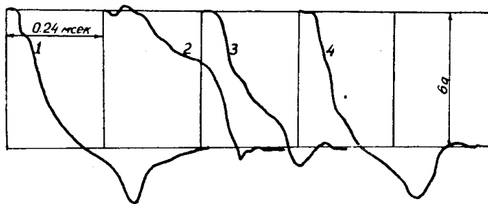
Рис. 3. Кривые тока коммутации в продольной цепи ЭМУ с шунтовой обмоткой при токе нагрузки 6а и частоте 50 гц.
