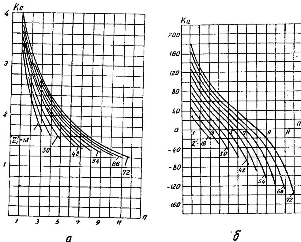
Рис. 2. К расчету усилий на изогнутые отрезки лобовых частей: а) геометрический фактор для расчета усилий притяжения к стали статора, б) геометрический фактор для расчета аксиальных усилий.
