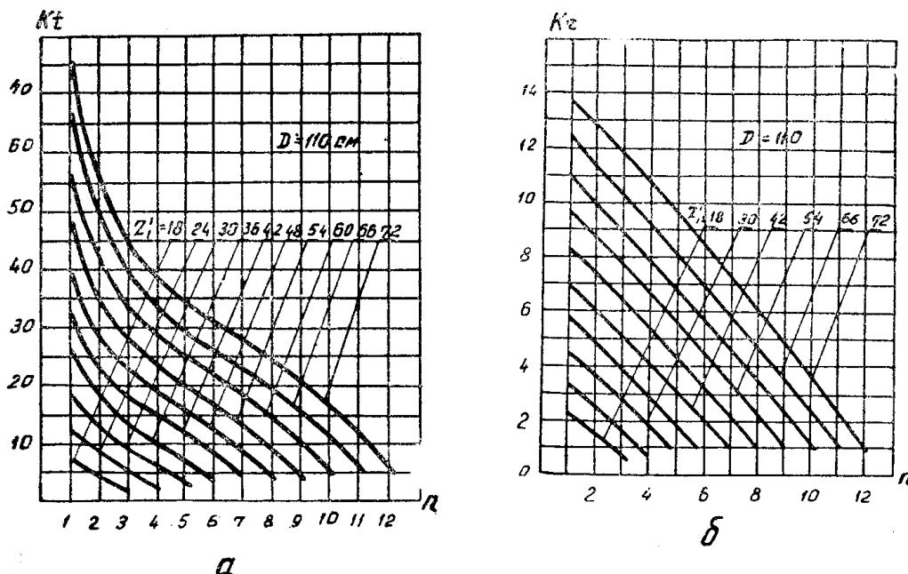
Рис. 1. К расчету усилий на прямолинейные отрезки лобовых частей:
