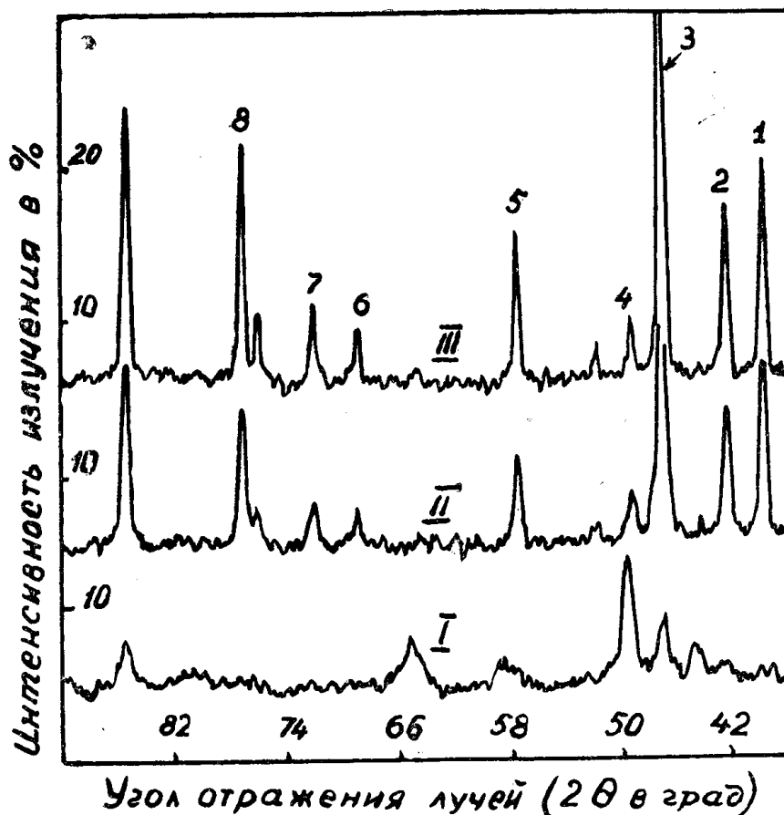
Рис. 1. Рентгенограмма I — для свежеприготовленного окисно-кобальтового катализатора, обработанного при 105°C. Рентгенограмма II — для образца \text{Co}_3\text{O}_4 , прокаленного при 550°C. Рентгенограмма III — для образца \text{Co}_3\text{O}_4 после испытания на каталитическую активность при температурном интервале 600—850°C.
