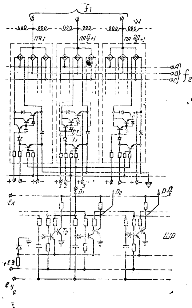
Рис. 3. Принципиальная электрическая схема рабочих ячеек и управления преобразователя частоты.
