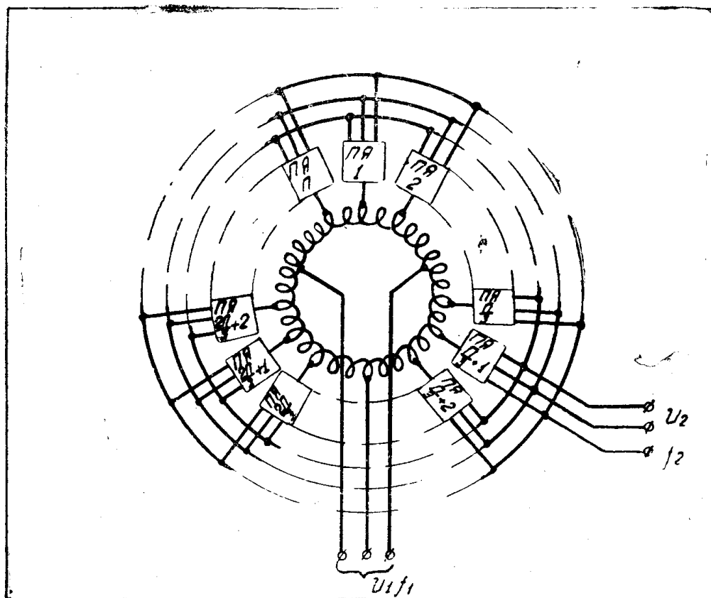
Рис. 2. Принципиальная схема преобразователя частоты с полупроводниковым коллектором.
