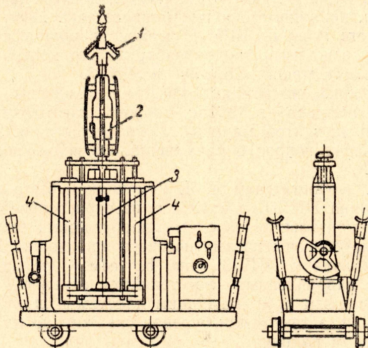
Рис. 4. Бурильно-роторная машина БРМ-1:
