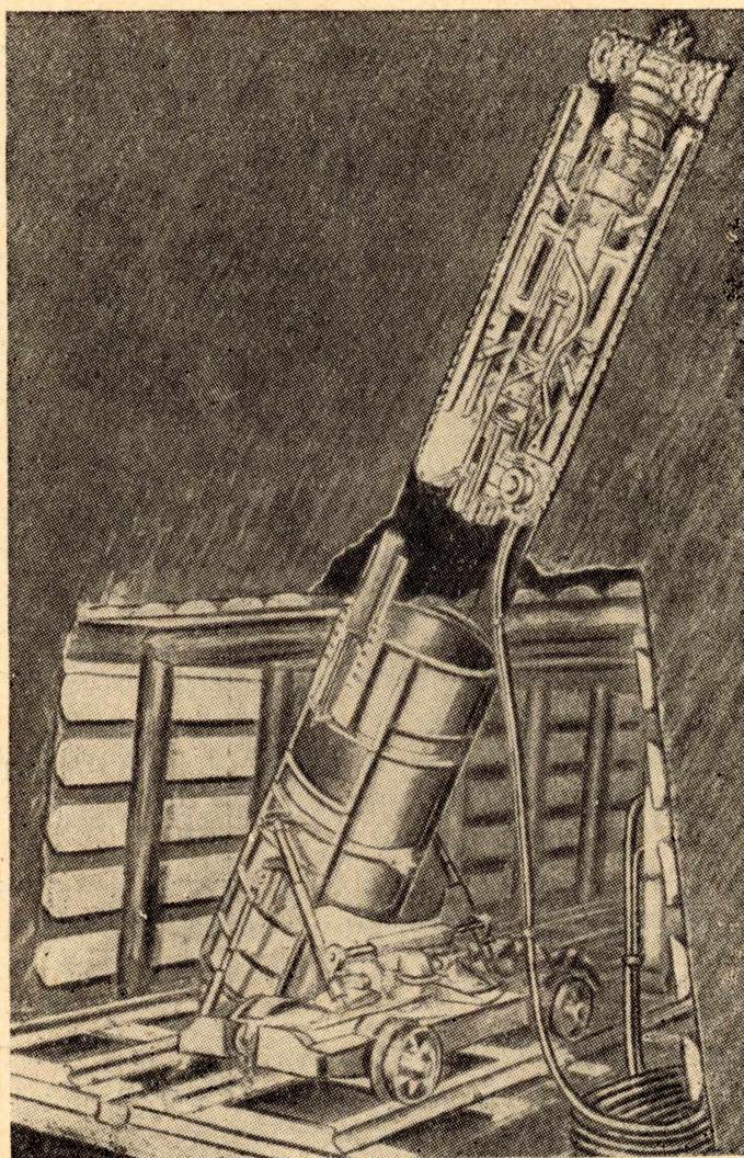
Рис. 5. Пневмопроходчик ППГ-3.
