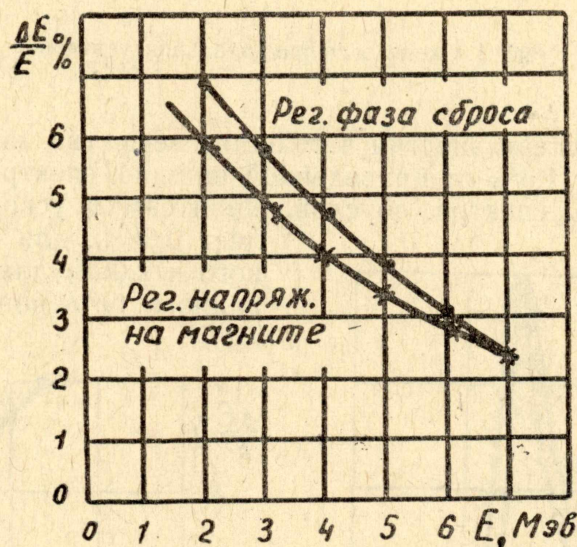
Рис. 4. Зависимость энергетического спектра от энергии при различных методах ее регу-
