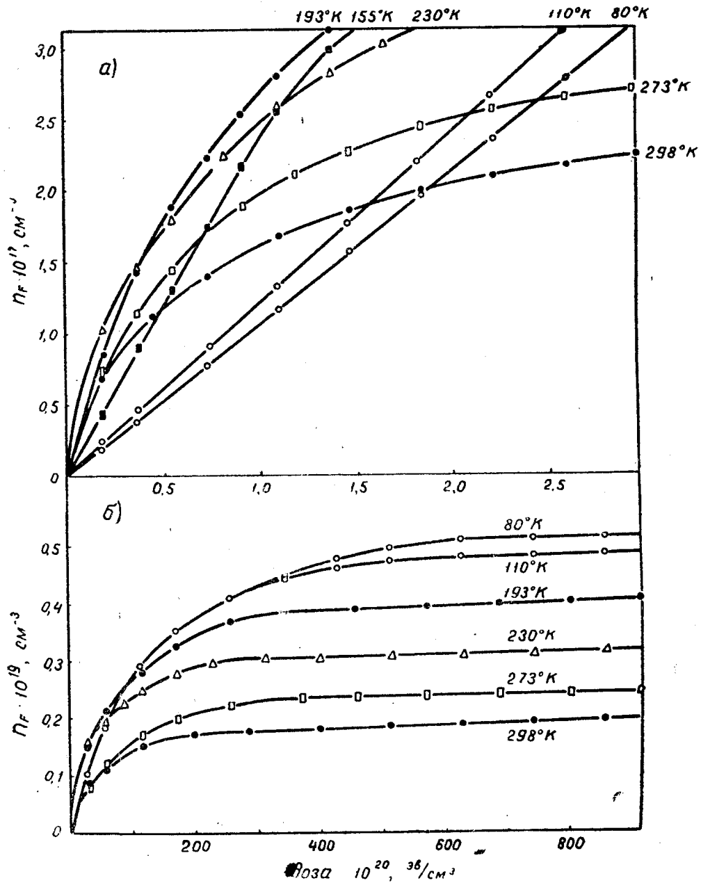
Рис. 3. Кинетика накопления F -центров в КСІ под действием протонов при различных температурах.
