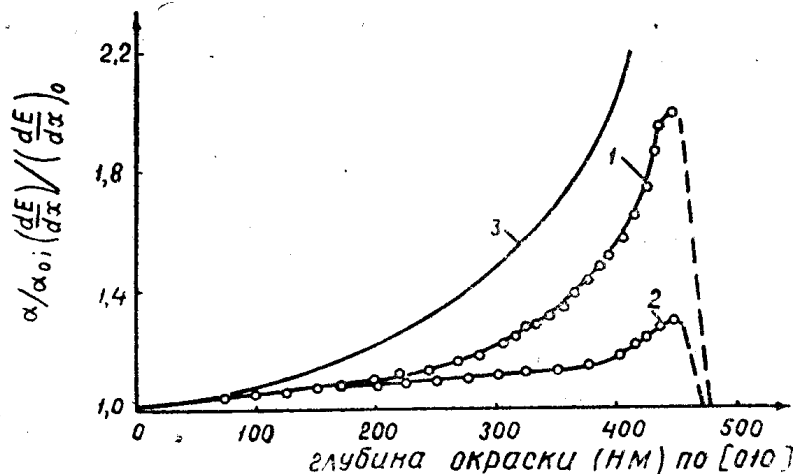
Рис. 2. Относительное распределение концентрации F-центров ( \alpha/\alpha_0 ) по глубине окрашенного протонами слоя кристалла KCl. Кривые 1 и 2 соответствуют дозам 3,75 \cdot 10^{12} и 7,5 \cdot 10^{13} протон. \text{см}^{-2} соответственно. Кривая 3 — относительное распределение удельных ионизационных потерь протонов в KCl, рассчитанное по данным работы [12]
