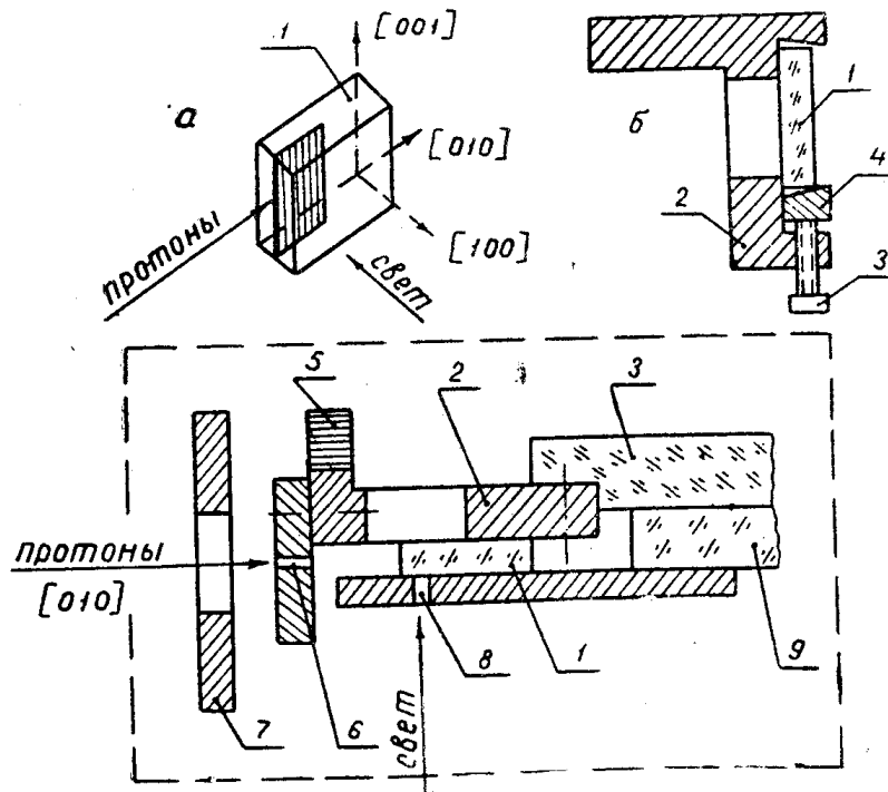
Рис. 1. Схема эксперимента
