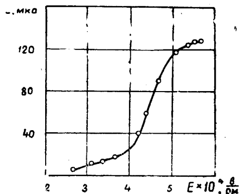
Рис. 4. Вольт-амперная характеристика для прессованного азид свинца. ( d = 150 мкн, P = 1600 атм)
