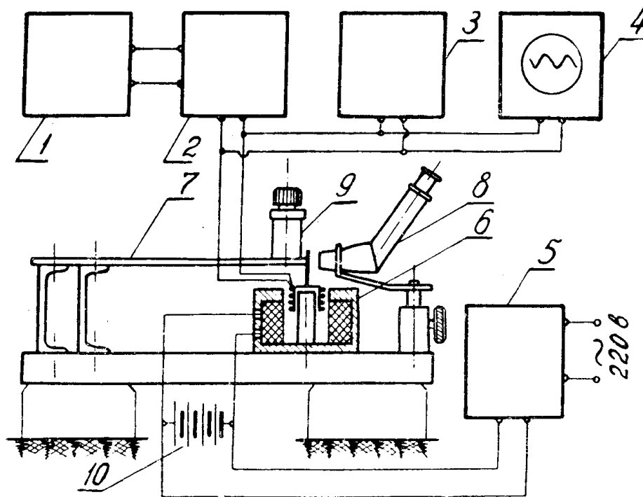
Рис. 2. Схема вибростенда с аппаратурой для тарировки вибродатчиков: 1 — звуковой генератор ЗГ-2А, 2 — электронный широкополосный усилитель, 3 — измеритель частоты ИЧ-6, 4 — катодный осциллограф ЭО-7, 5 — селеновый двухполупериодный выпрямитель АВС-5, 6 — электродинамический вибратор, 7 — упругая балка, 8 — микроскоп, 9 — вибродатчик, 10 — аккумулятор, 11 — массивная чугунная плита с опорами.
