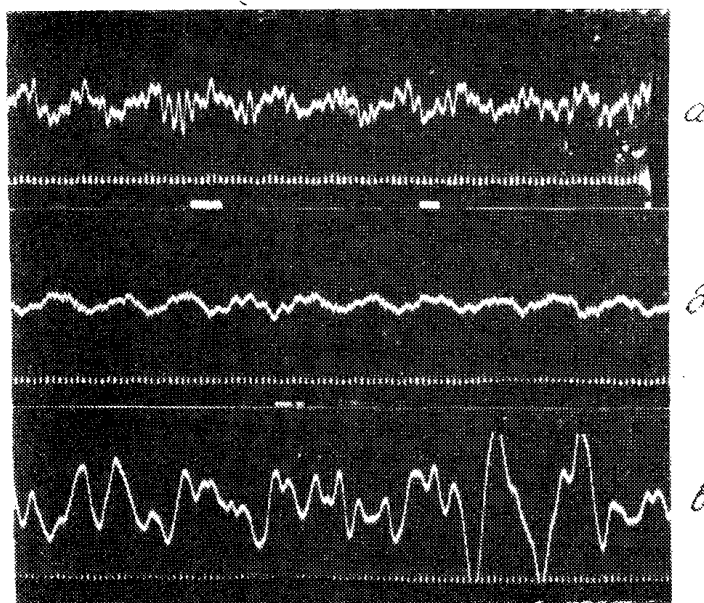
Рис. 3. Вибрации рабочих мест в различных точках около виброплатформ типа СМ-476 с длинной рамой: а) вибрации пола цеха около электромотора-вибратора у края виброплатформы, б) вибрации пола цеха около середины рамки виброплатформы, в) вибрации тонкого металлического листа, закрывающего с торцов колодец виброплатформы.
