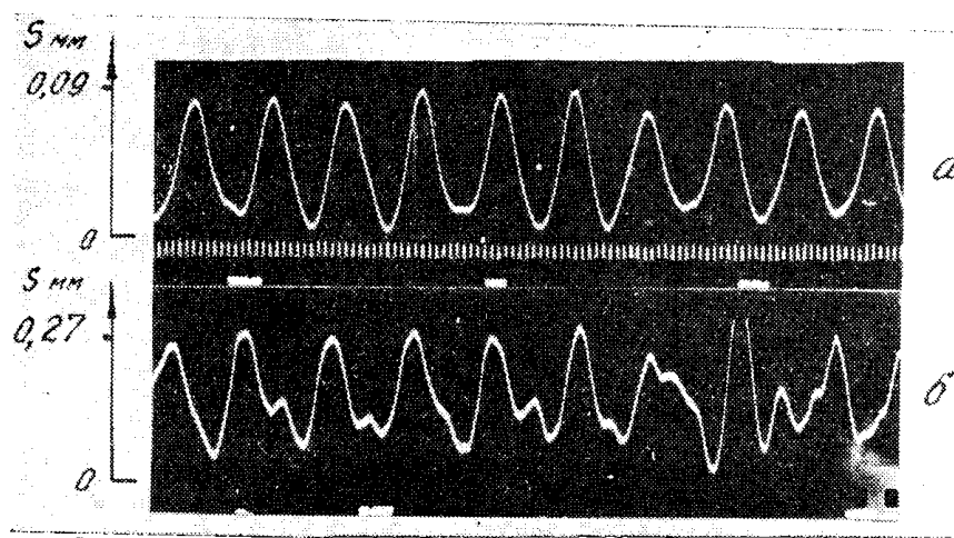
Рис. 5. Вибрации рамы бетоноукладчика: а) бункер с бетоном, б) бункер без бетона.
