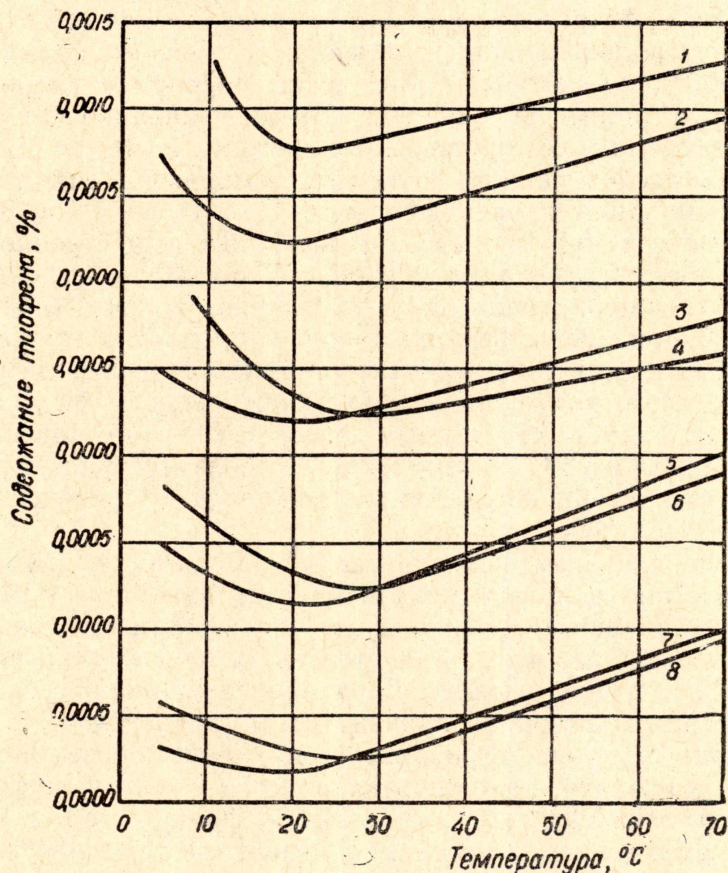
Рис. 1. Зависимость содержания тиафена в бензоле от температуры процесса очистки при различных временах перемешивания БТФ с формалином: 1—в присутствии кислой смолки, \tau_{\text{пер}}=5 мин.; 2—без кислой смолки, \tau_{\text{пер}}=5 мин.; 3—без кислой смолки, \tau_{\text{пер}}=10 мин.; 4—в присутствии кислой смолки, \tau_{\text{пер}}=10 мин.; 5—без кислой смолки, \tau_{\text{пер}}=20 мин.; 6—в присутствии кислой смолки, \tau_{\text{пер}}=20 мин.; 7—без кислой смолки, \tau_{\text{пер}}=30 мин.; 8—в присутствии кислой смолки, \tau_{\text{пер}}=30 мин.
