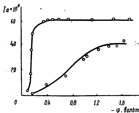
Рис. 1. Зависимость глубины анодного зубца Bi и Cu от потенциала накопления 1,5 НСl; C_{\text{Cu}} - C_{\text{Bi}} = 0,15 ; V = 2 \text{ мл} ; \tau = 2 \text{ мин} ; r_{\text{к}} = 0,04 \text{ см} .
