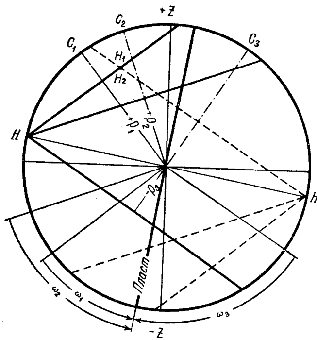
Рис. 1. Геометрическая форма связи между ориентировкой скважин, видимыми углами падения слоев в кернах и элементами залегания горных пород.
